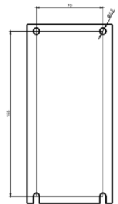
Розмітка монтажних отворів (мм)
